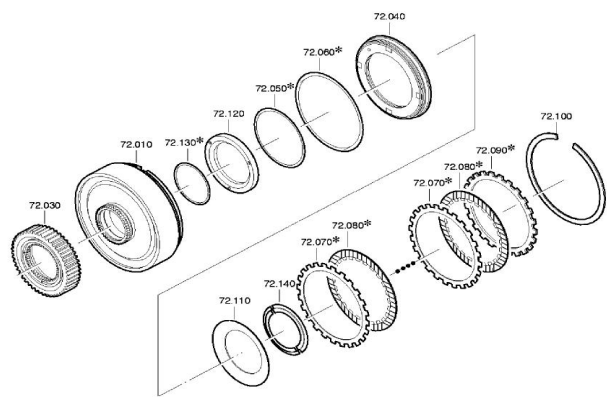
Clutch B
